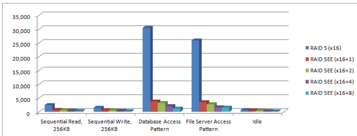
图表 17 RAID 5 和 RAID 5EE 的图表
